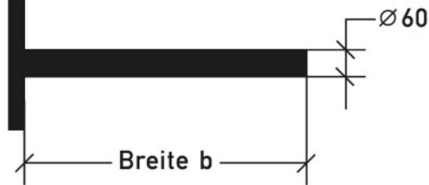
U-Profil für Bandbefestigung
